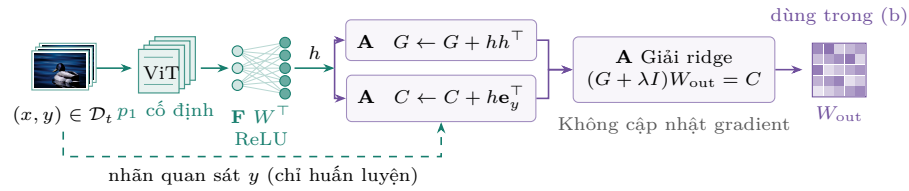
Hình 1. Vòng đời tham số và hợp nhất hai tầng. (a) Quy trình PET kế thừa huấn luyện bộ điều hợp/các đầu, không huấn luyện mạng xương sống. (b) Mọi mô-đun đều cố định: Tầng 1 sửa đề xuất DRM; Tầng 2 đặt cổng cho hợp nhất lớp bằng \ell . Một vector điểm RP phục vụ cả hai tầng. (c) Dữ liệu huấn luyện hiện tại cập nhật giải tích G, C, W_{\text{out}} với p_1, W cố định. Chỉ các lớp/tác vụ đã thấy tham gia. Ảnh và cột chỉ minh họa, không phải dự đoán đo được. Ảnh: T. G. Barnes/USFWS (phạm vi công cộng).
