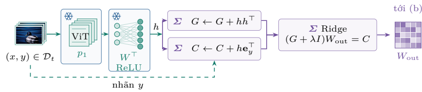
Hình 1. Vòng đời tham số và hợp nhất hai tầng. (a) Huấn luyện các mô-đun PET hiện tại. (b) Điểm RP cố định s sửa đề xuất tác vụ DRM và hỗ trợ hợp nhất lớp có cổng biên. (c) Dữ liệu tác vụ hiện tại cập nhật G, C, W_{\text{out}} bằng ridge dạng đóng, không phát lại dữ liệu hay cập nhật gradient.
