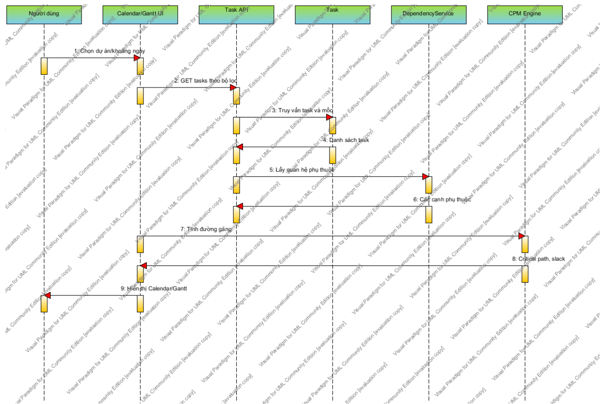
Hình 3-29 Sơ đồ sequence SEQ10 – Lịch và Gantt
