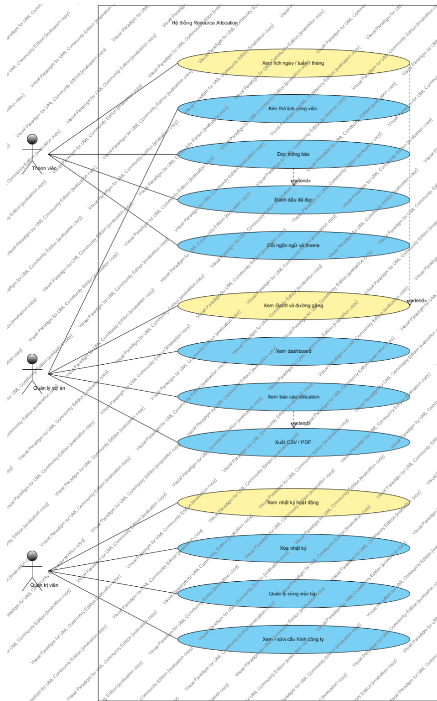
Hình 3-9 Sơ đồ use case phân hệ Lịch, báo cáo, thông báo và cấu hình
