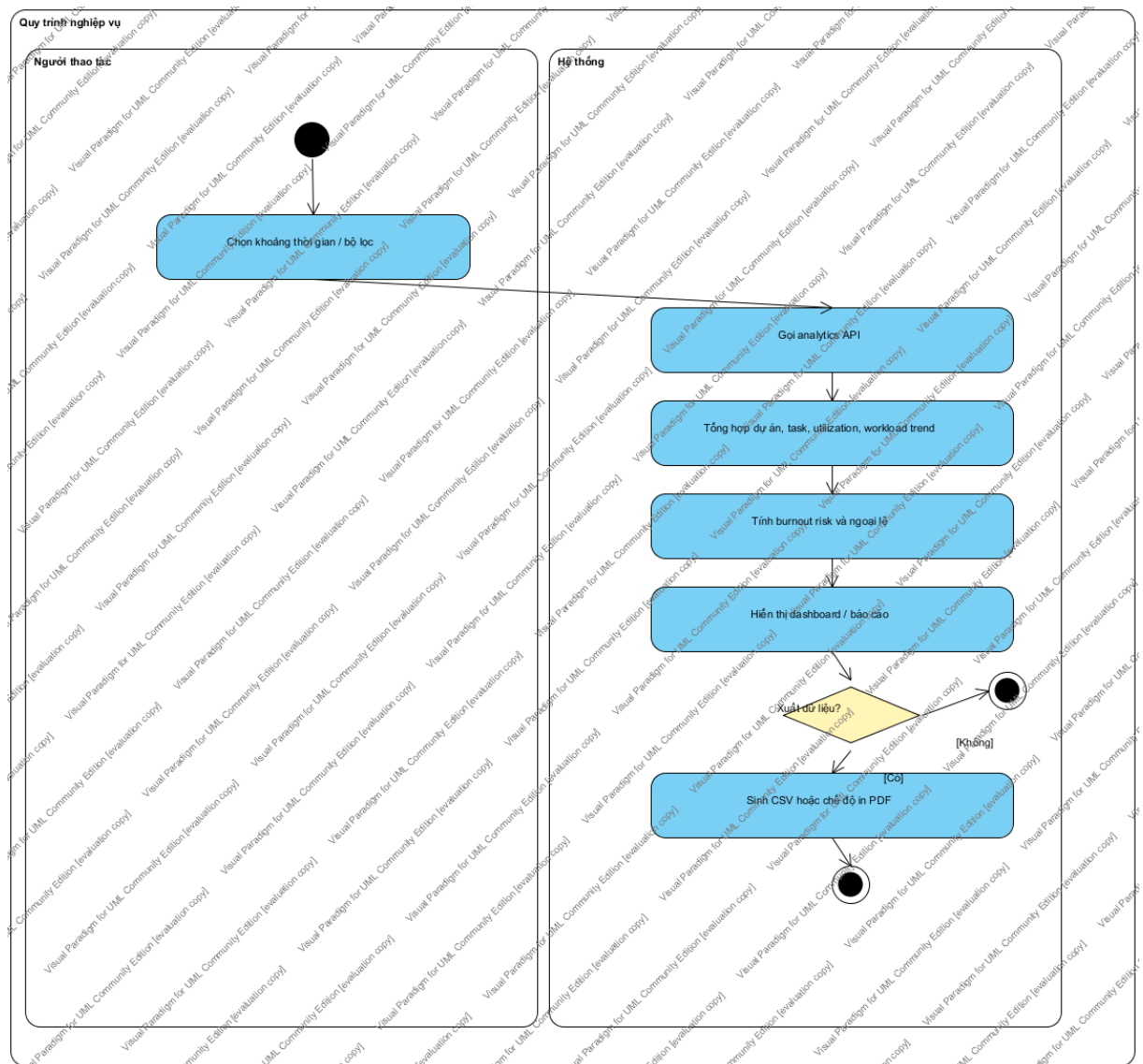
Hình 3-27 Sơ đồ activity ACT10 – Báo cáo và xuất dữ liệu
