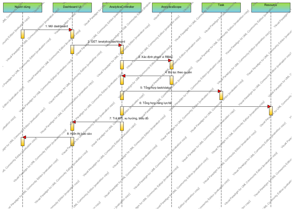
Hình 3-28 Sơ đồ sequence SEQ09 – Tải dashboard và báo cáo
