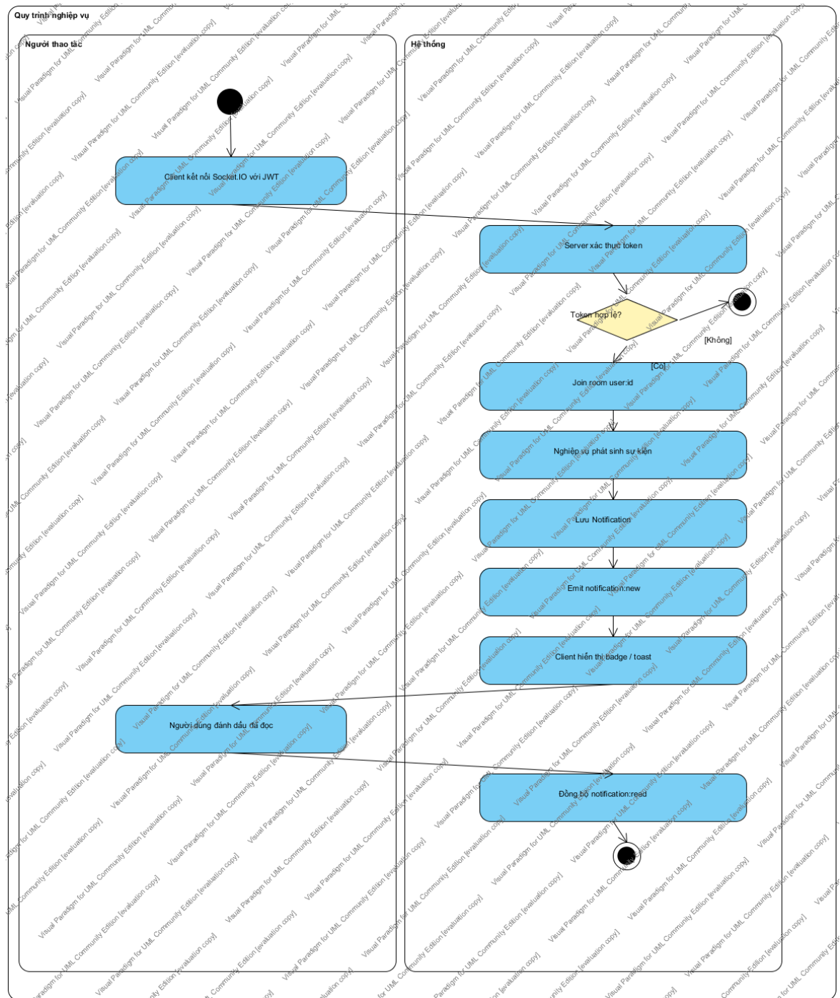
Hình 3-23 Sơ đồ activity ACT08 – Thông báo thời gian thực
