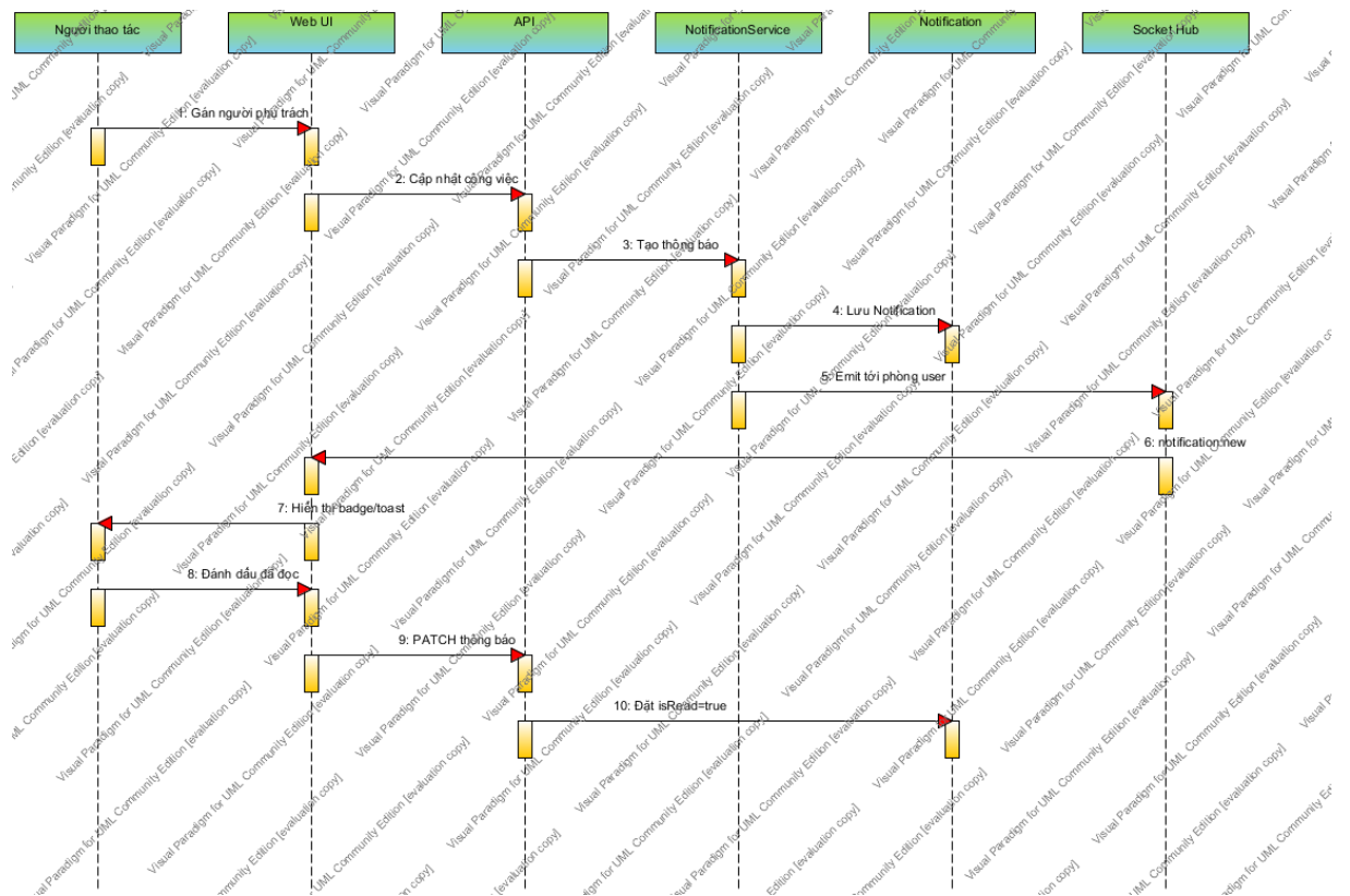
Hình 3-24 Sơ đồ sequence SEQ03 – Thông báo thời gian thực
