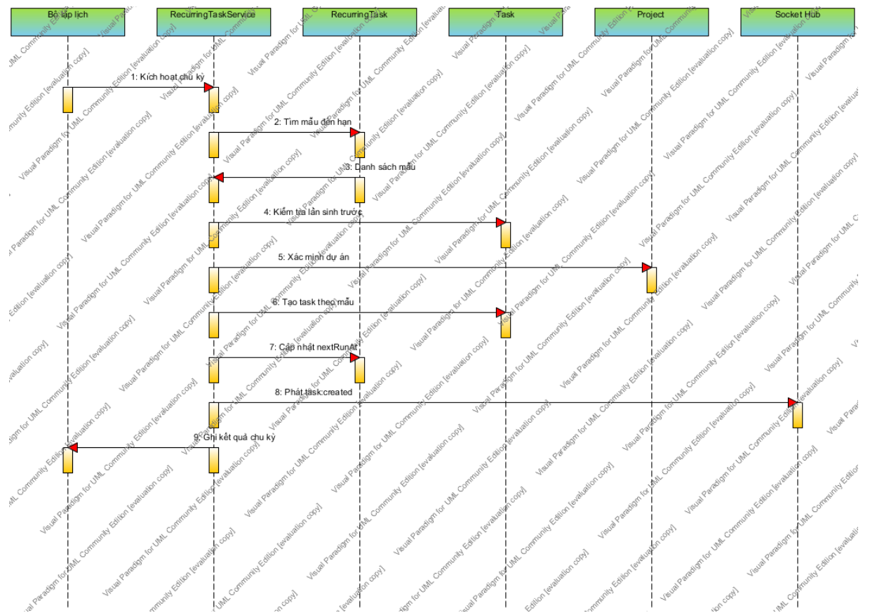
Hình 3-22 Sơ đồ sequence SEQ08 – Sinh công việc lặp
