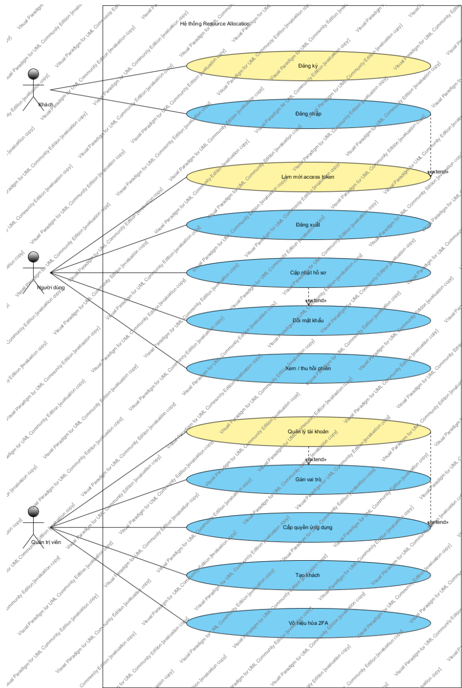
Hình 3-5 Sơ đồ use case phân hệ Xác thực, tài khoản và phân quyền
