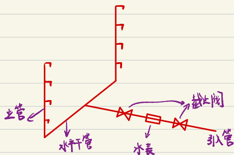
直接供水: (无水箱)
