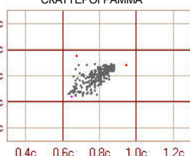
СКАТТЕРОГРАММА
