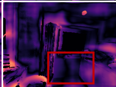
Mismatch (Ours)
