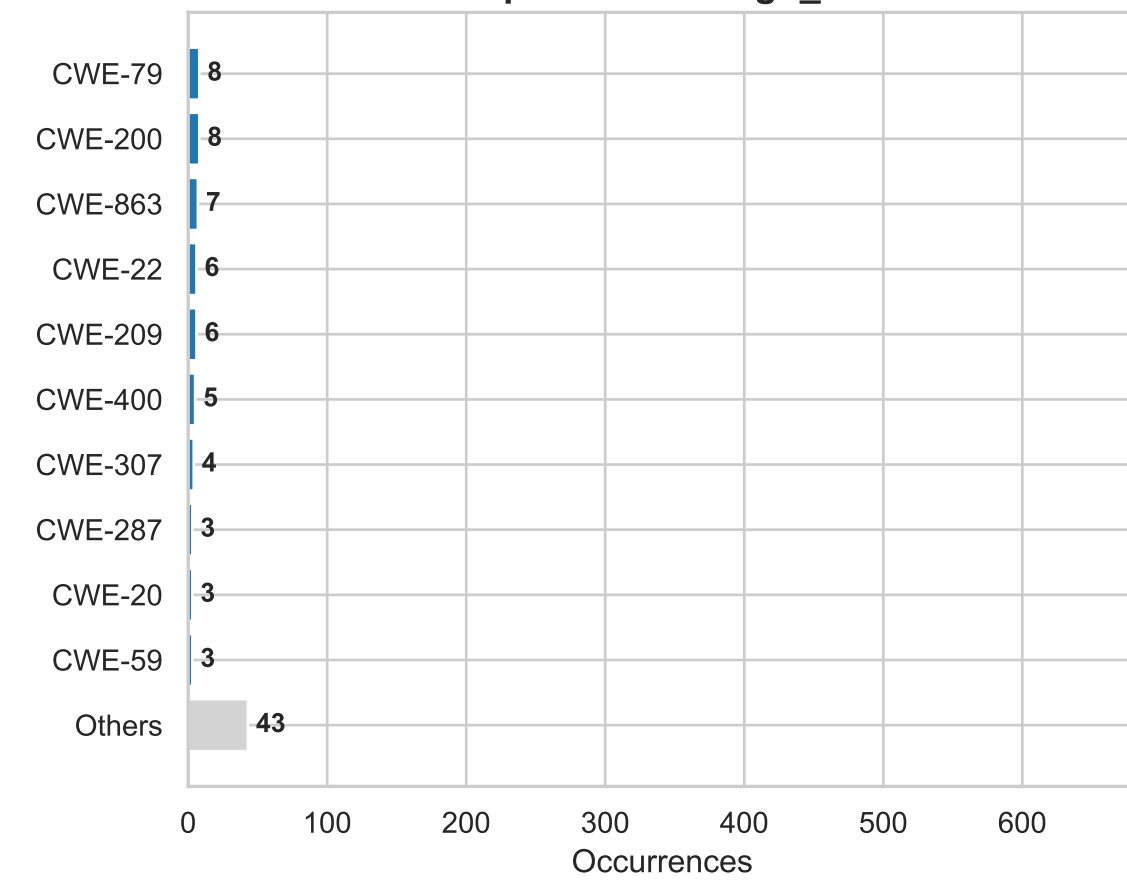
Top 10 CWEs: gitlab
