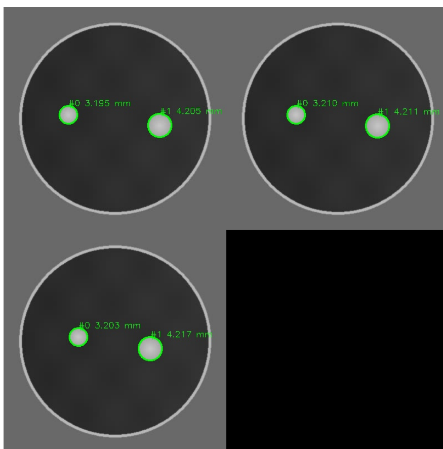
Рис. 3: Контрольные кадры с найденными окружностями, идентификаторами и измеренными диаметрами.
