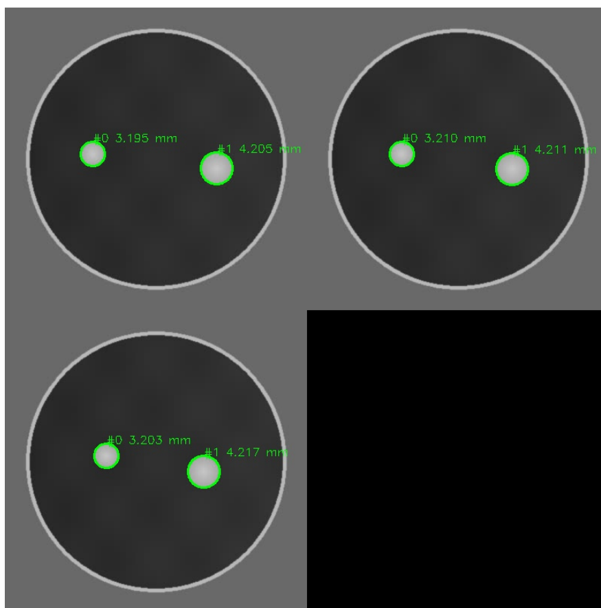
Рис. 2: Контрольные кадры с найденными окружностями, идентификаторами и измеренными диаметрами.
