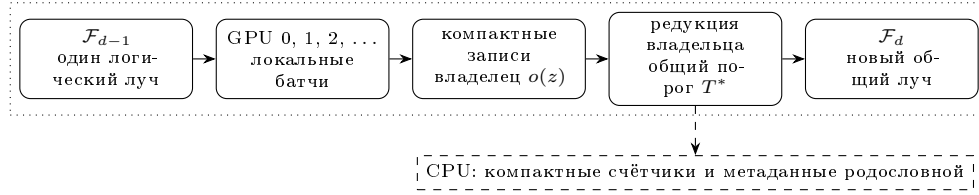
Рис. 2: Один глобальный луч физически распределён по GPU. Одинаковые ключи поступают одному владельцу; порог и финальный \text{top-}B относятся ко всему множеству кандидатов, без семантических локальных квот. Сплошные стрелки обозначают GPU hot data, пунктирная — только компактные метаданные на CPU.
