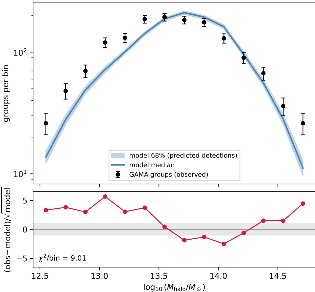
Posterior predictive (Nessie mock)
