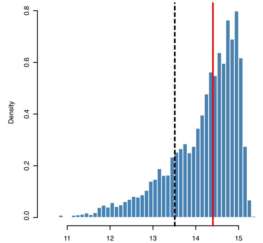
M_{*} posterior
