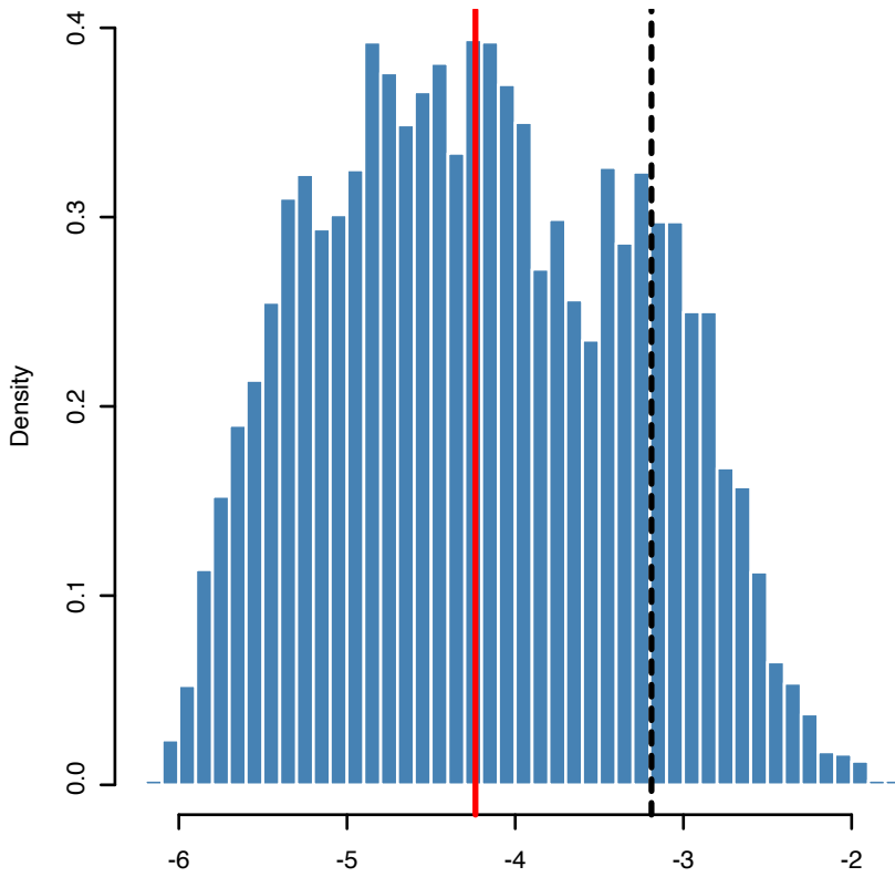
\log_{*} posterior
