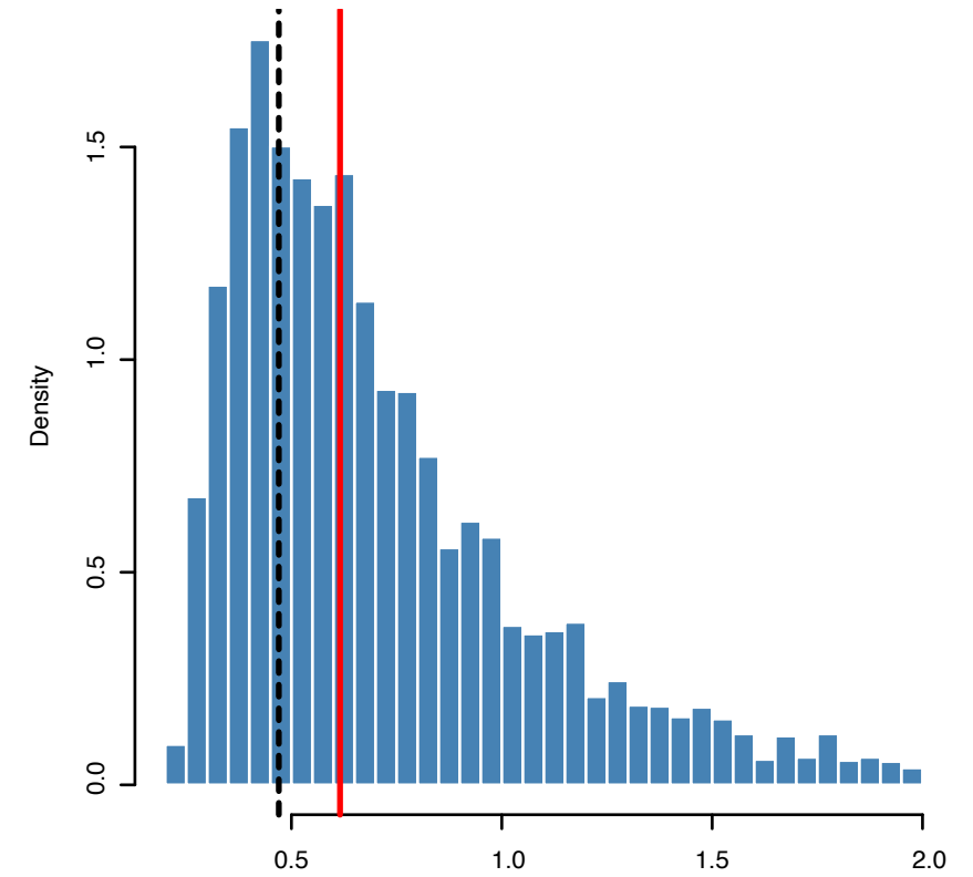
\beta posterior
