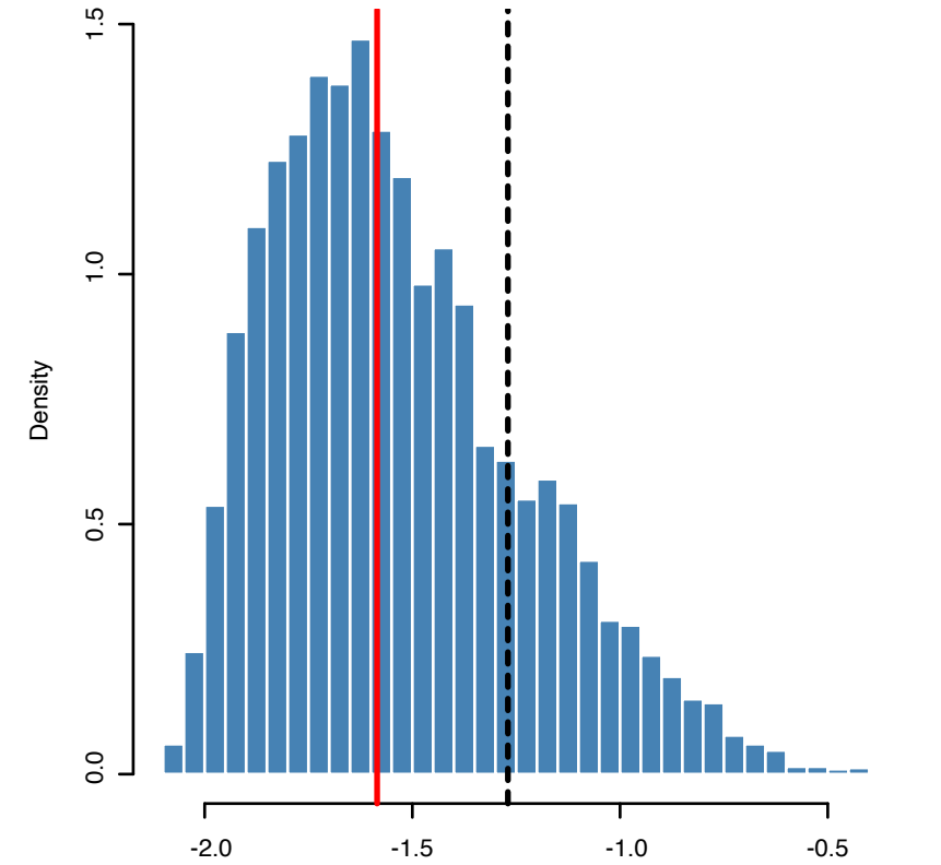
\alpha posterior
