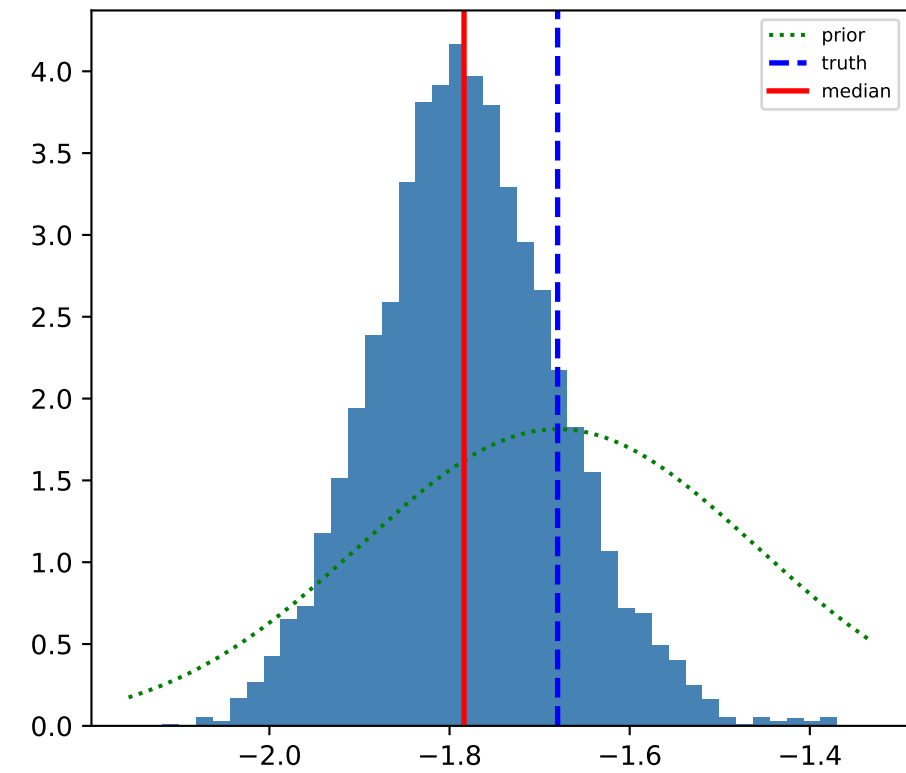
\alpha
