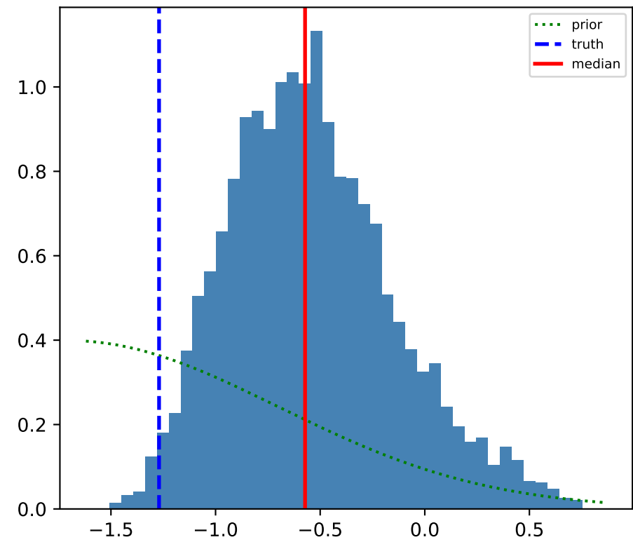
\alpha
