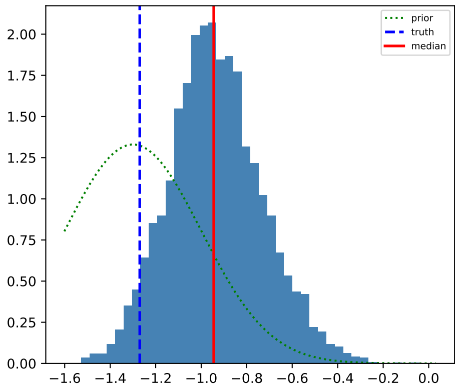
\alpha
