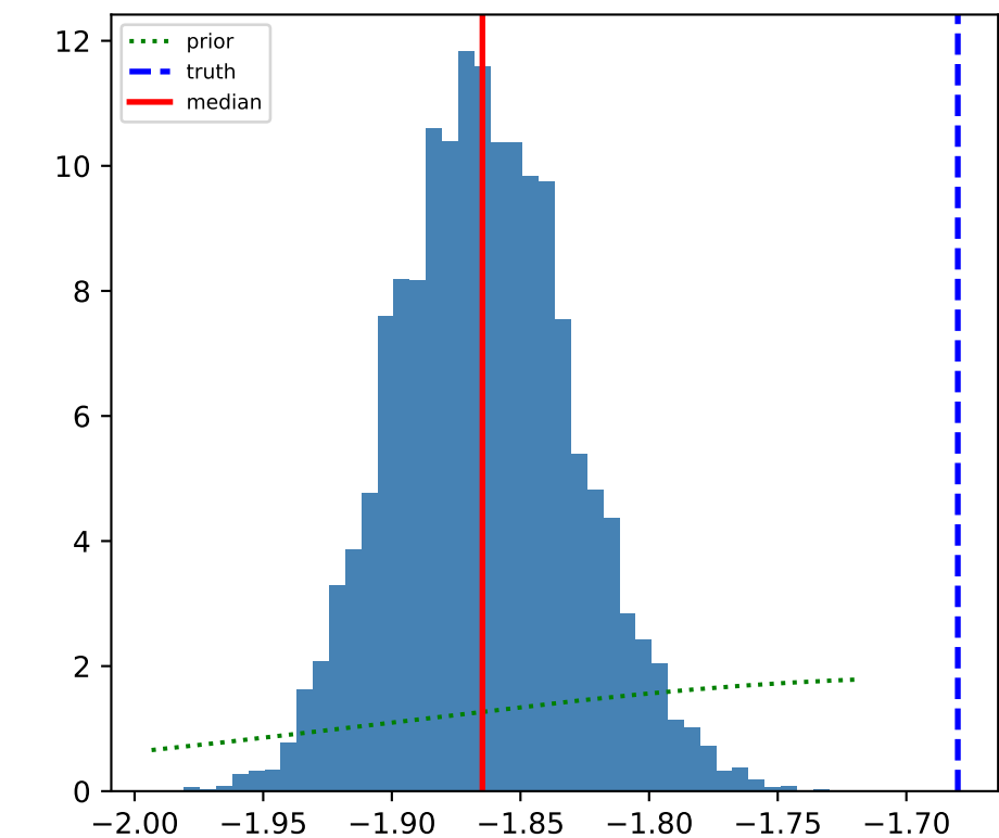
\alpha
