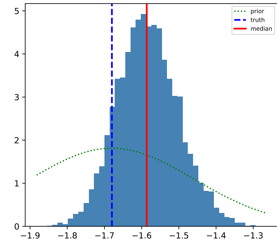
\alpha
