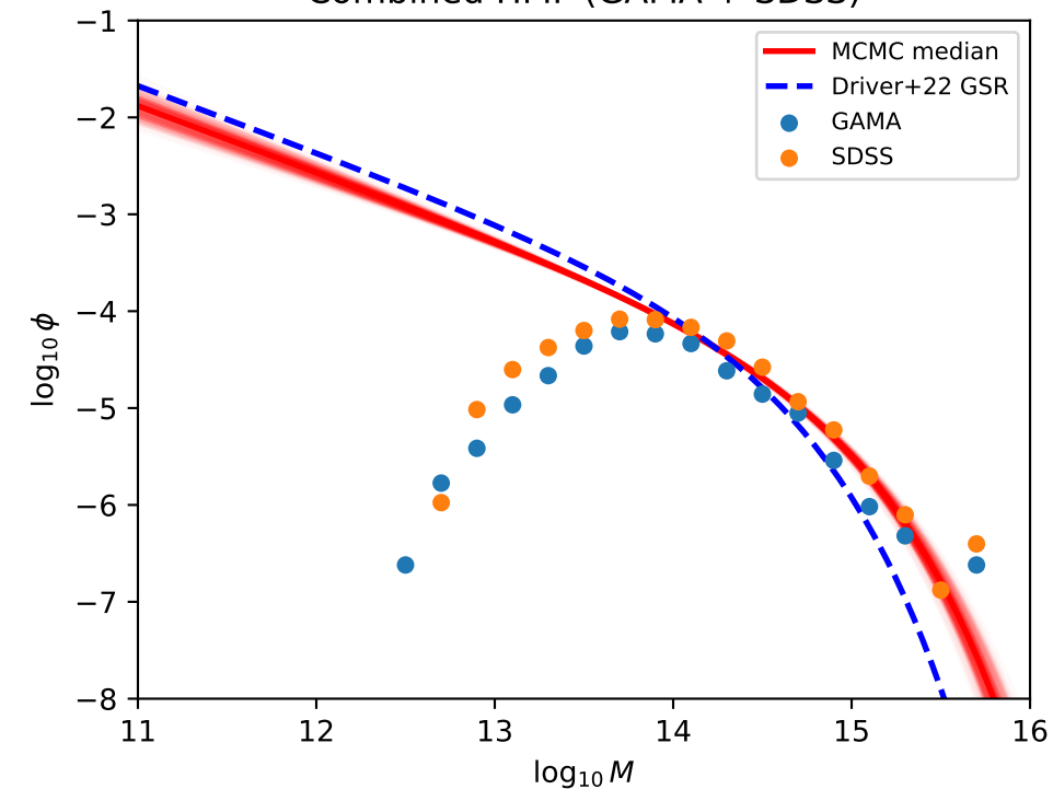
\alpha
