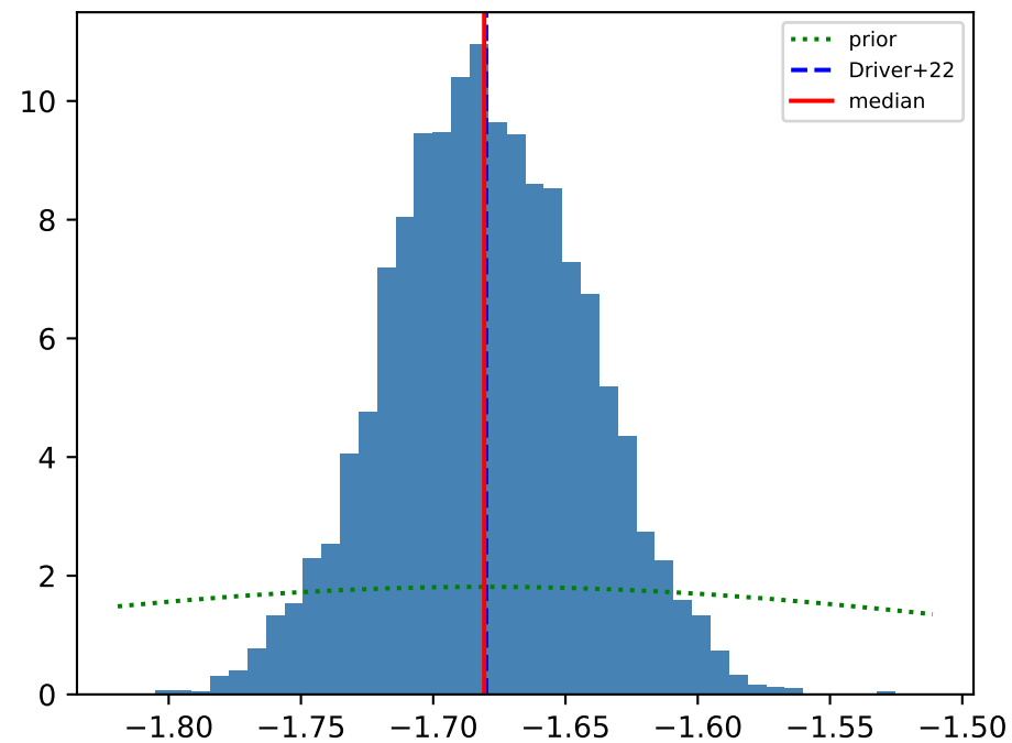
\alpha
