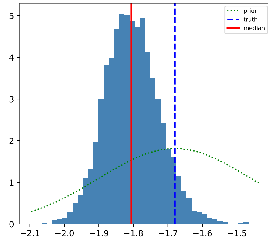
\alpha
