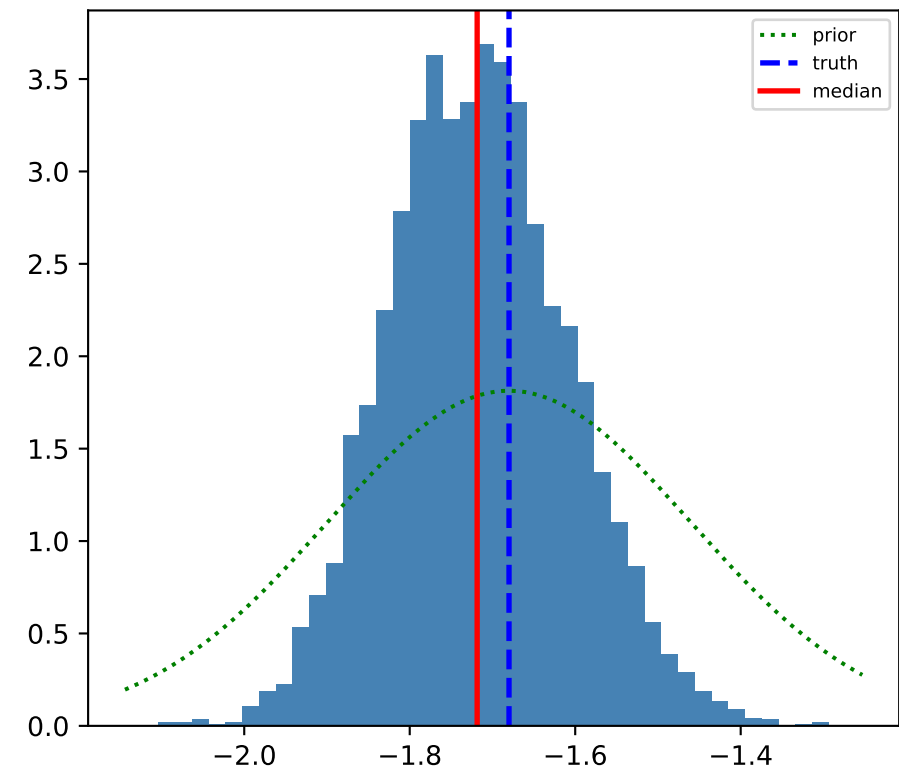
\alpha
