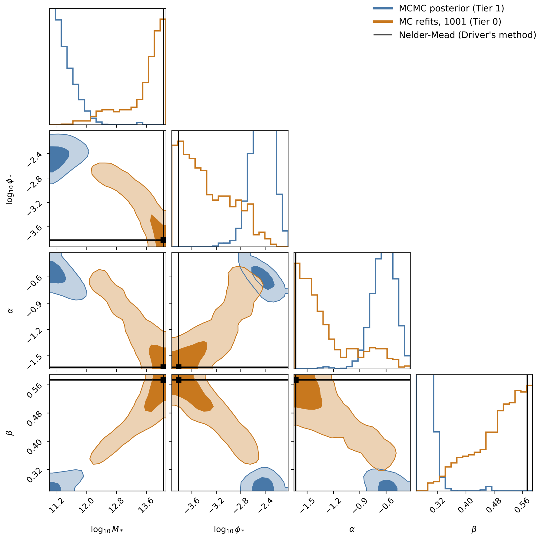
GS: MRP posterior vs Driver's Monte-Carlo refits
