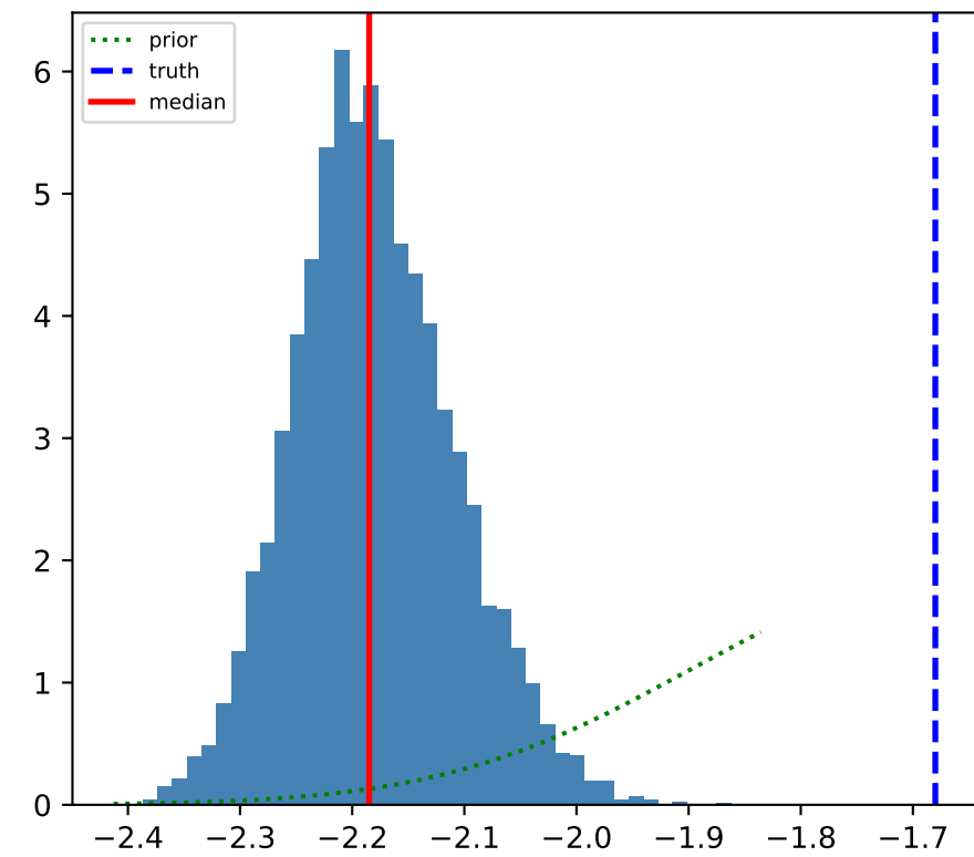
\alpha
