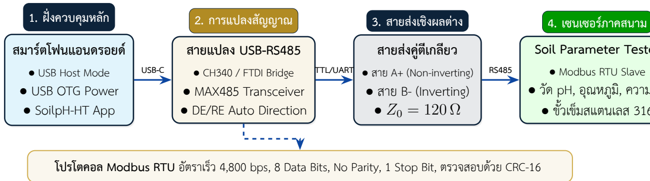
ภาพที่ 2.1 ฟังก์ชันการเชื่อมต่อทางกายภาพและการไหลของสัญญาณดิจิทัลผ่านพอร์ต USB Type-C OTG สู่หัววัด Soil Parameter Tester
