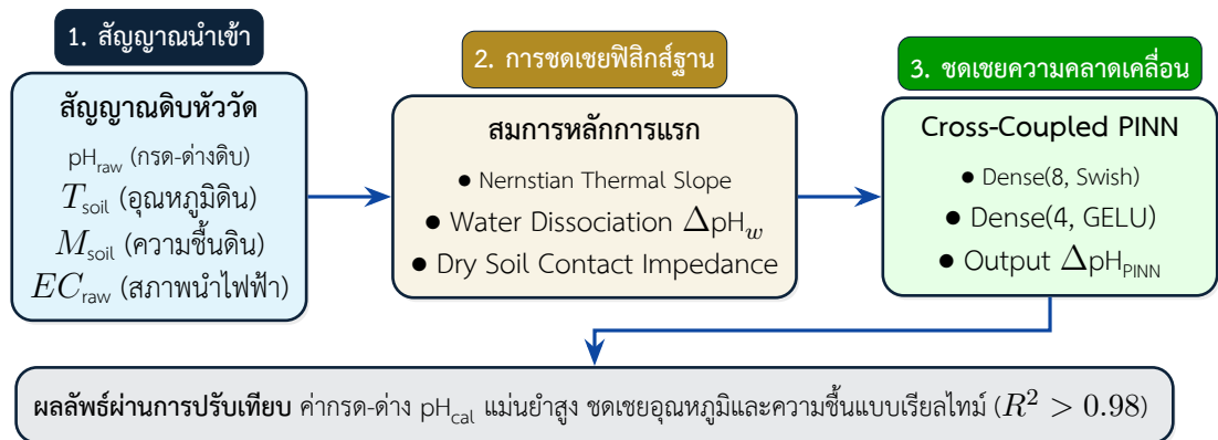
ภาพที่ 3.1 ผังสถาปัตยกรรมโครงข่ายประสาทเทียมอิงฟิสิกส์ (PINN) และกระบวนการขดเซยสองขั้นตอนแบบเรียลไทม์สำหรับวิเคราะห์ค่ากรด-ด่างดิน
