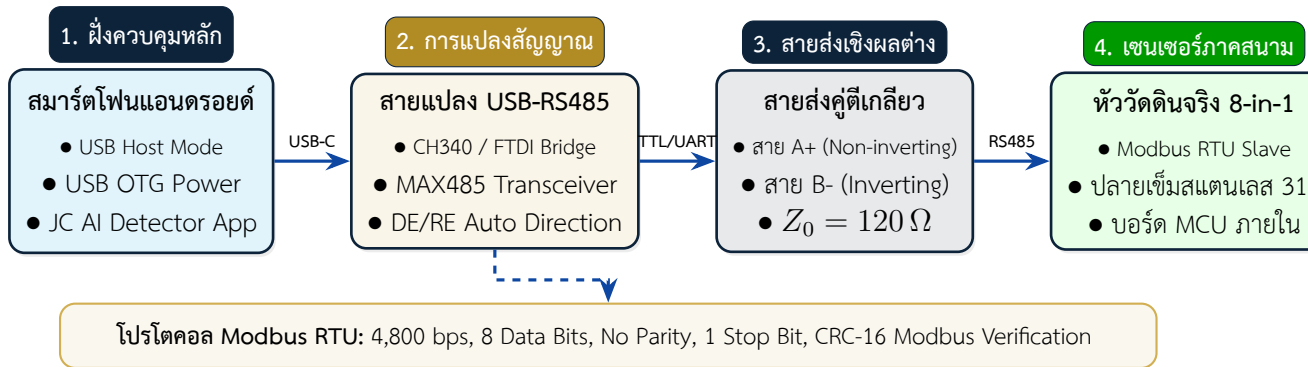
ภาพที่ 2.1 ฟังก์ชันการเชื่อมโยงทางกายภาพและการไหลของสัญญาณดิจิทัลผ่านพอร์ต USB Type-C OTG สู่หัววัดดินจริง
