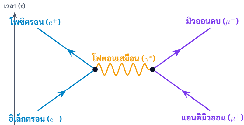
ภาพที่ 3.4 แผนภาพไฟน์แมนแสดงการประลัยคู่อิเล็กตรอน-โพซิตรอนกลายเป็นคู่มิวออน ( e^- + e^+ \rightarrow \gamma^* \rightarrow \mu^- + \mu^+ )
