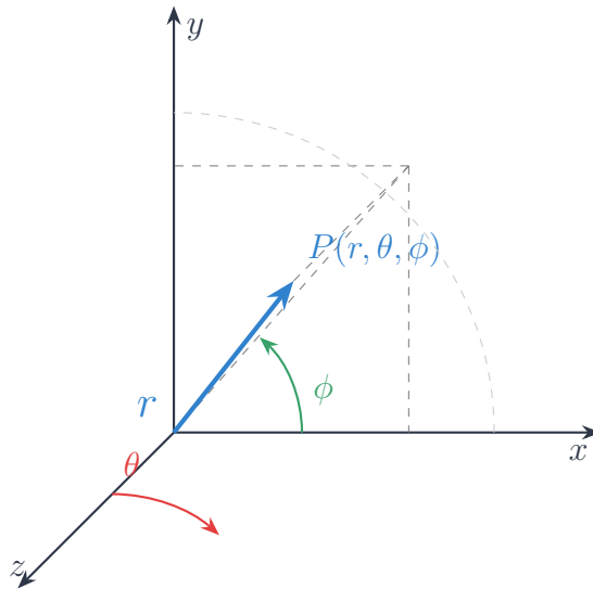
ภาพที่ 1.2 ระบบพิกัดทรงกลม (r, \theta, \phi) แสดงมุมเชิงขั้ว \theta และมุมทิสราบ \phi
