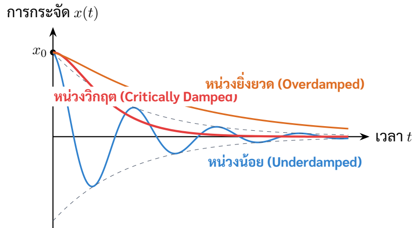
ภาพที่ 9.1 เปรียบเทียบพฤติกรรม การเคลื่อนที่ของ ระบบการสั่น หน่วง 3 รูปแบบ: หน่วงยิ่งยวด (Overdamped), หน่วงวิกฤต (Critically Damped) และหน่วงน้อย (Underdamped)
