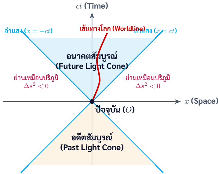
ภาพที่ 1.2 แผนภาพกรวยแสง (Light Cone) แสดงโครงสร้างการส่งผ่านผลเชิงเหตุและผล (Causality) ในปริภูมิ-เวลายามินคอฟสกี
