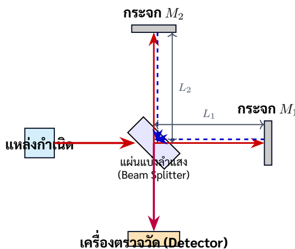
ภาพที่ 1.1 ผังการทดลองของไมเคิลสัน-มอร์ลีย์ (Michelson-Morley Experiment) ซึ่งแสดงผลลัพธ์เป็นศูนย์
