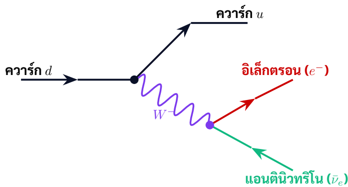
ภาพที่ 3.2 แผนภาพไฟน์แมนแสดงการสลายตัวบีตาลบในระดับควาร์ก ( d \rightarrow u + W^- \rightarrow u + e^- + \bar{\nu}_e )
