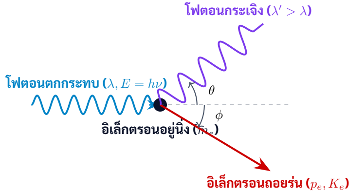
ภาพที่ 2.1 แผนภาพการกระเจิงคอมป์ตัน (Compton Scattering) แสดงการอนุรักษ์พลังงานและโมเมนตัมของโฟตอนกับอิเล็กตรอน
