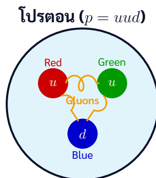
ภาพที่ 3.1 แบบจำลองโครงสร้างควาร์กและกลูออนภายในโปรตอน แสดงสมดุลประจุสี (Color Neutrality)
