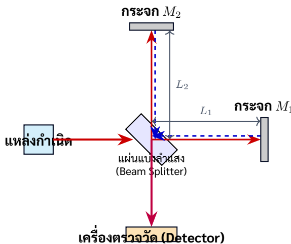
ภาพที่ 1.1 แผนผังการทดลองของไมเคิลสัน-มอร์ลีย์ (Michelson-Morley Experiment) ซึ่งแสดงผลลัพธ์เป็นศูนย์
