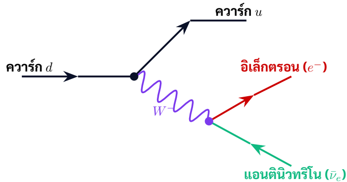
ภาพที่ 3.3 แผนภาพไฟน์แมนแสดงการสลายตัวบีตาในระดับควาร์ก ( d \rightarrow u + W^- \rightarrow u + e^- + \bar{\nu}_e )
