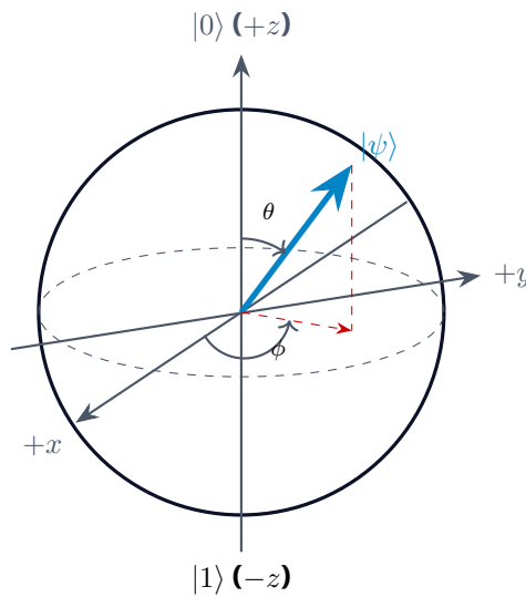
ภาพที่ 6.1 การแทนสถานะของคิวบิตบนทรงกลมบ্লอค (Bloch Sphere Representation)
