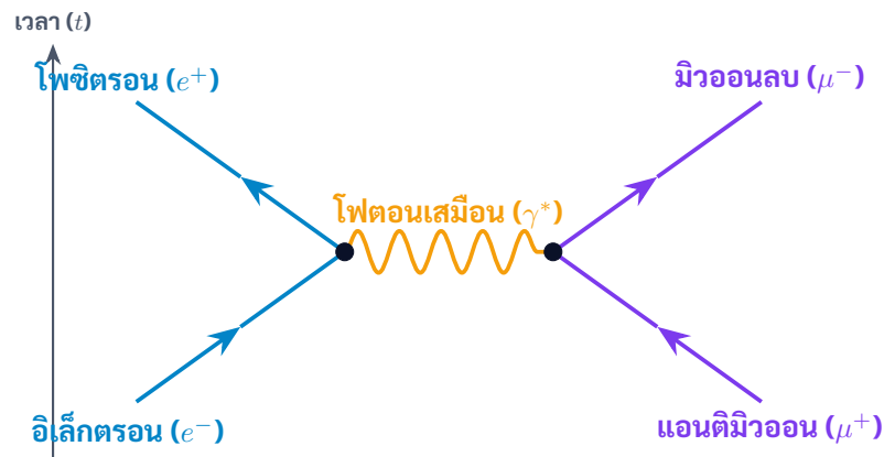
ภาพที่ 4.4 แผนภาพไฟน์แมนแสดงการประลัยคู่อิเล็กตรอน-โพซิตรอนกลายเป็นคู่มิวออน ( e^- + e^+ \rightarrow \gamma^* \rightarrow \mu^- + \mu^+ )
