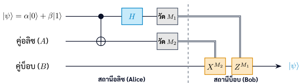
ภาพที่ 6.3 ผังวงจรควอนตัมเทเลพอร์ต (Quantum Teleportation Circuit) ถ่ายโอนสถานะ |\psi\rangle ไปยังปลายทาง
