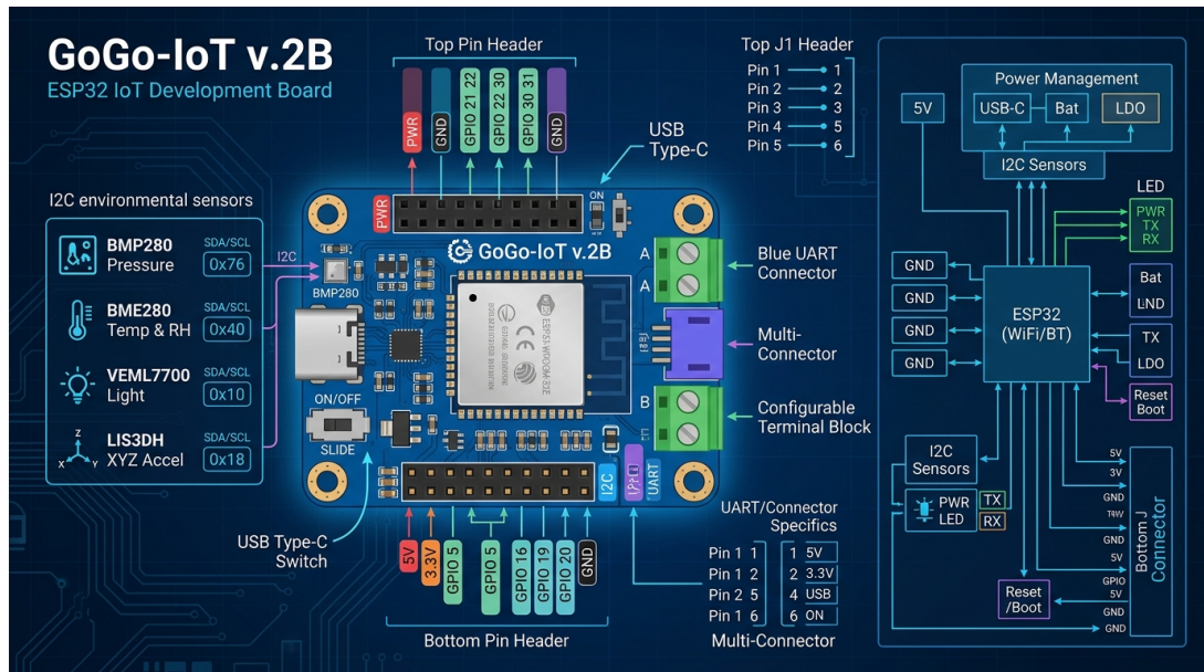
ภาพที่ 2.1 แผนผังกำหนดขาและบล็อกไดอะแกรมวงจรของบอร์ด GoGo-IoT v.2B (Schematic & Virtual Pinout Architecture)
