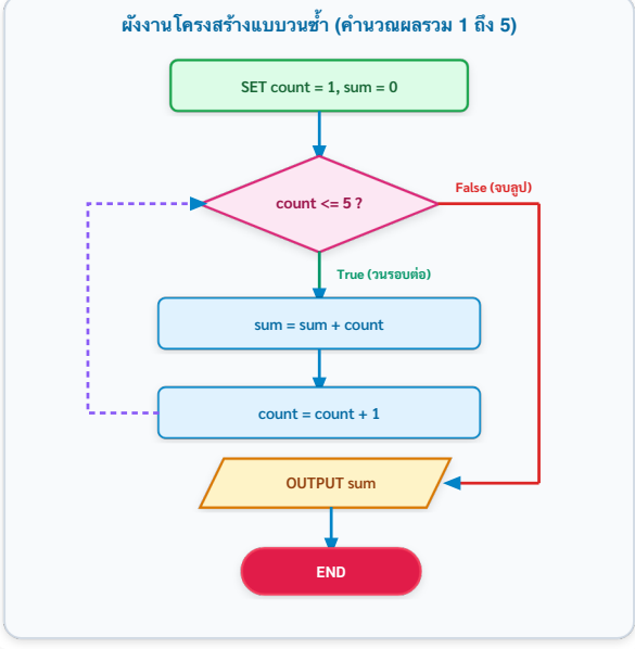
ภาพที่ 2.6 ผังงานโครงสร้างแบบวนซ้ำ การคำนวณผลรวมอนุกรมเลขคณิต 1 ถึง 5
