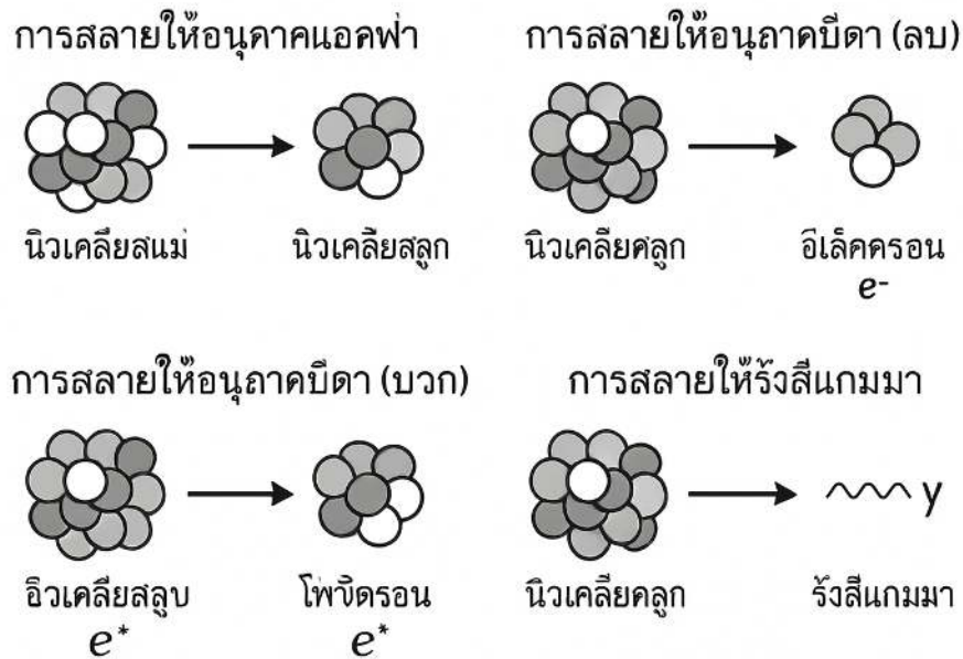
ภาพที่ 6.2 การสลายของนิวเคลียสกัมมันตรังสี
