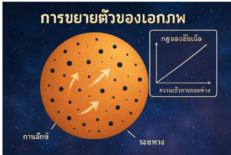
ภาพที่ 8.1 การขยายตัวของเอกภพและกฎของฮับเบิล
