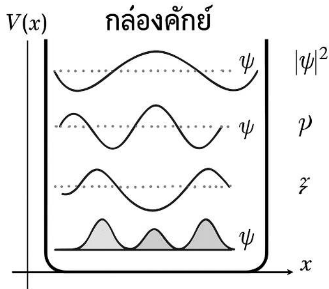
ภาพที่ 4.2 อนุภาคในกล่องศักย์
