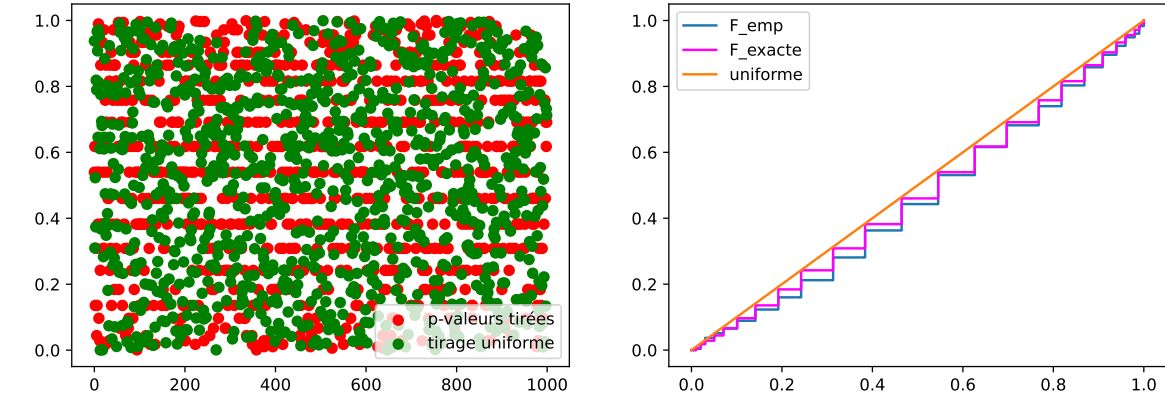
Figure 4: Répartition de 1000 p-valeurs comparées avec 1000 tirages d’une loi uniforme (gauche) et comparaison entre la fonction de répartition théorique et empirique des p-valeurs sous conditionnement (droite).
