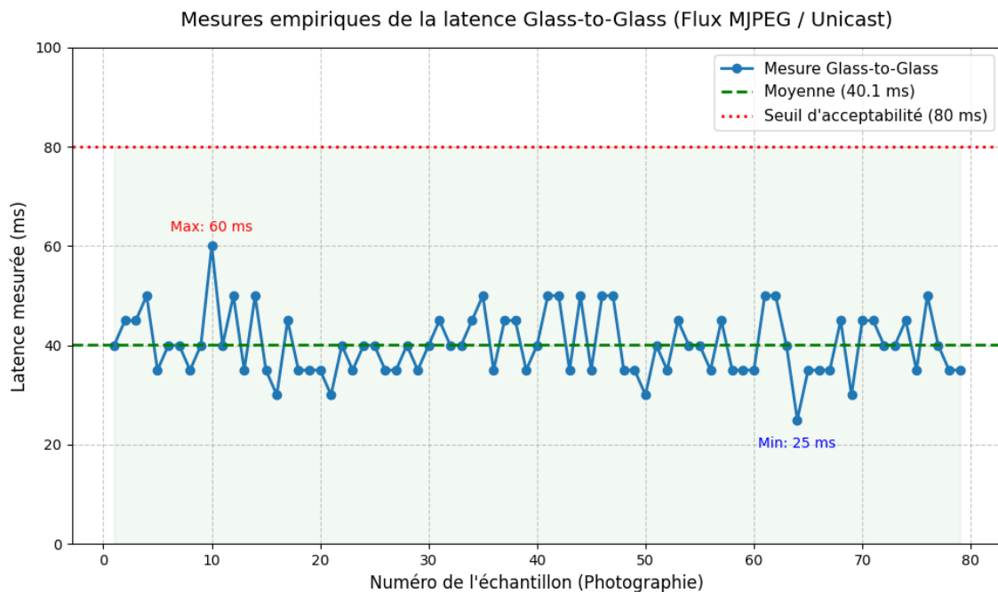
FIGURE 21 – Graphique de l'analyse statistique des 79 mesures réelles de latence Glass-to-Glass (Unicast MJPEG @ 60 FPS)
