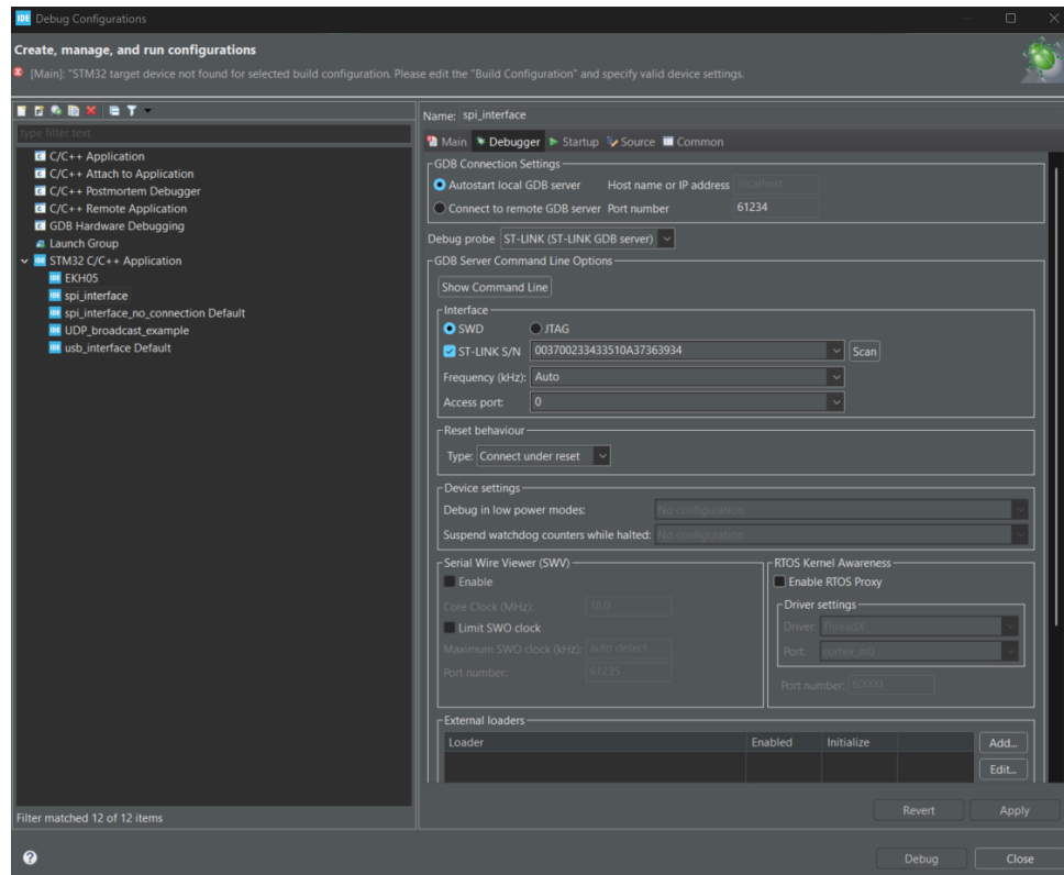
FIGURE 7 – Configuration du serveur GDB ST-LINK dans STM32CubeIDE
