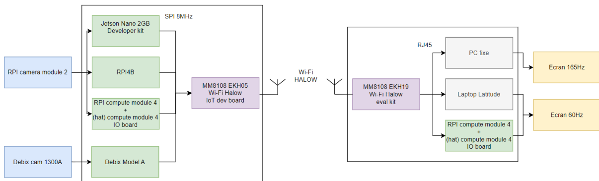
FIGURE 4 – Architecture globale du système de transmission vidéo avec les différentes options testées
