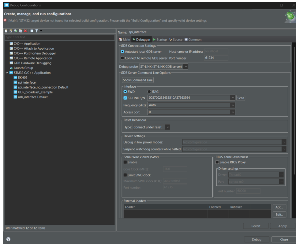
FIGURE 5 – Configuration du serveur GDB ST-LINK dans STM32CubeIDE
