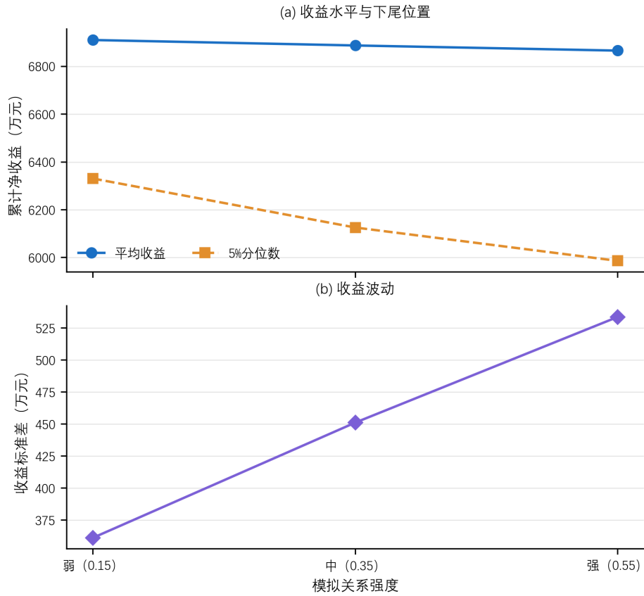
图 6 问题三模拟关系强度的收益敏感性
