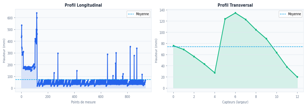
Figure 1 — Profil longitudinal (gauche) et profil transversal (droite) de la surface analysee.
