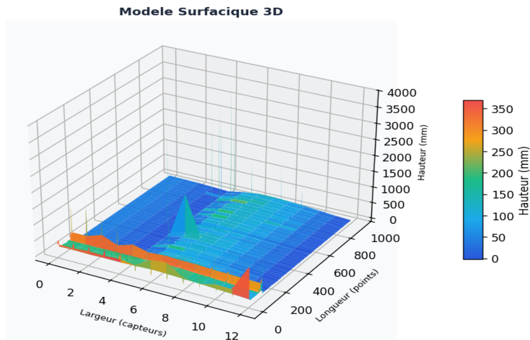
Figure 3 — Representation tridimensionnelle de la surface routiere. Le dégradé de couleur indique les niveaux de hauteur (bleu = bas, rouge = haut).
