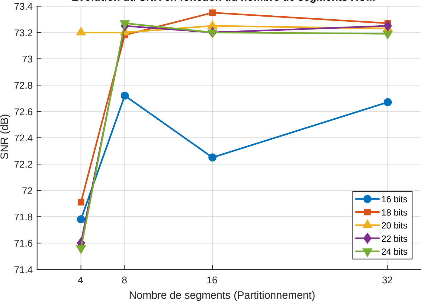
Evolution du SNR en fonction du nombre de segments ROM
