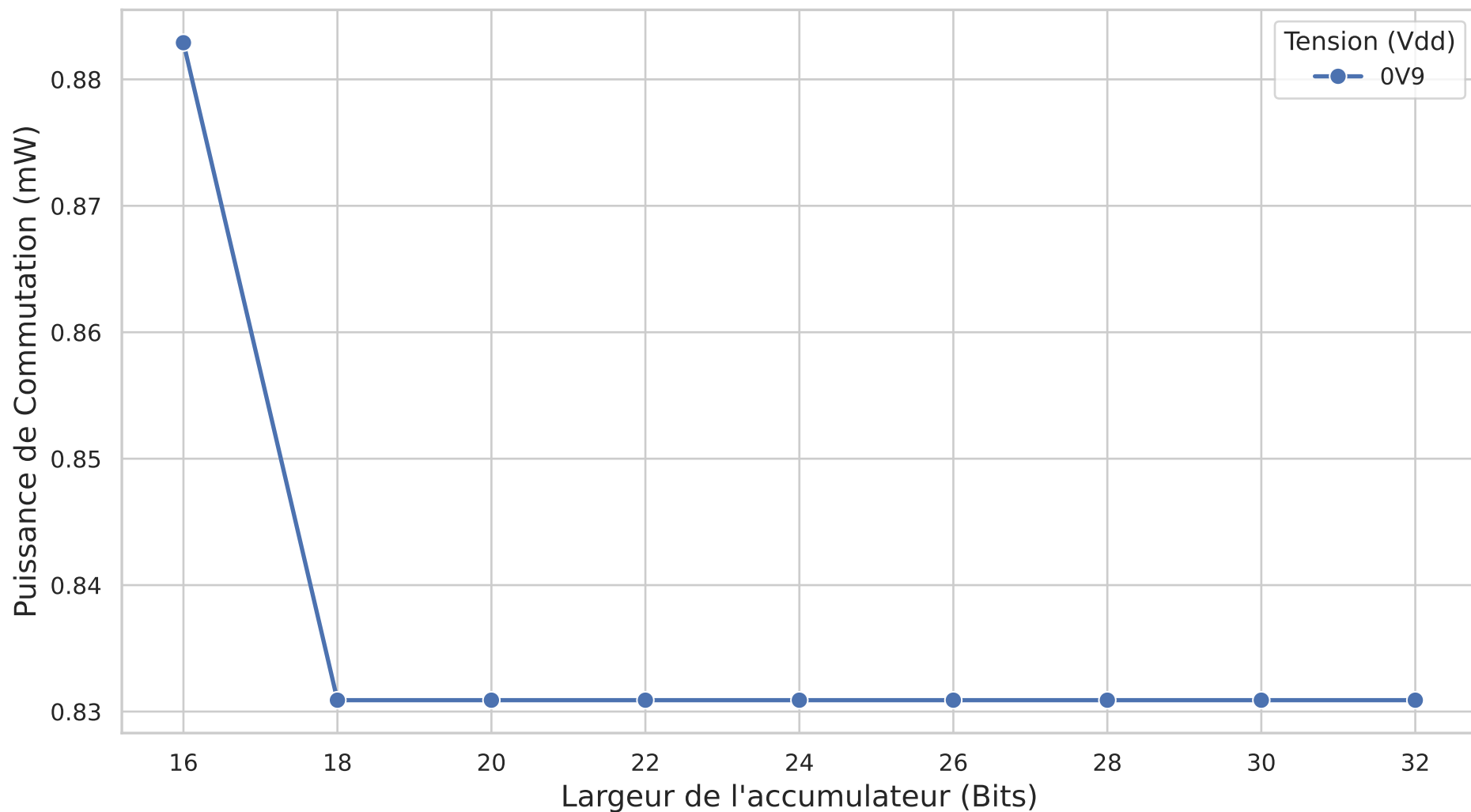
Puissance de commutation (dissipee dans les interconnexions)
