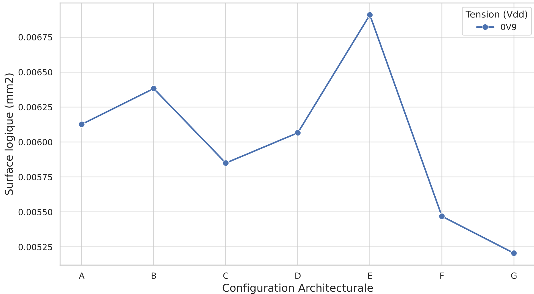
Empreinte silicium par configuration
