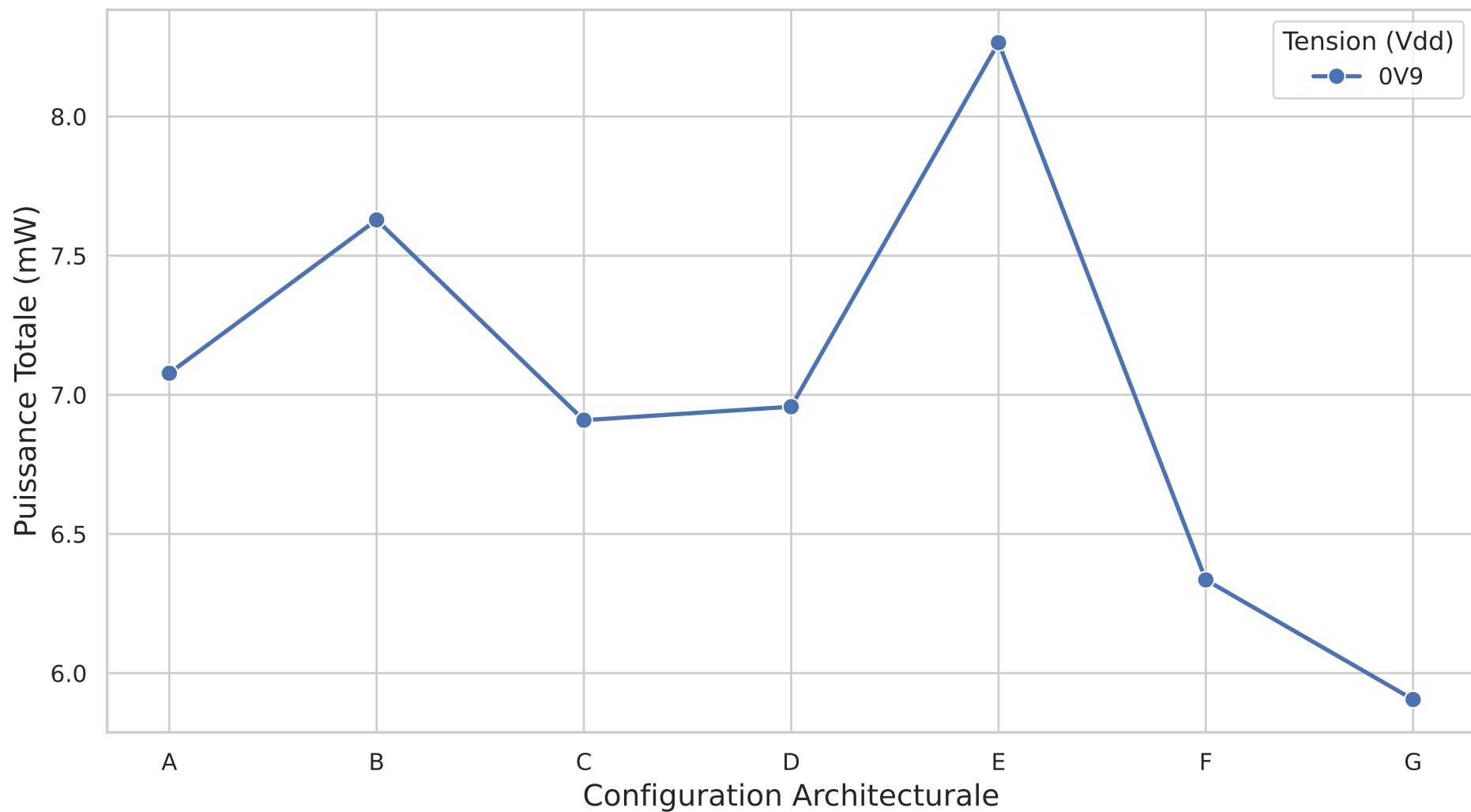
Consommation energetique totale par configuration
