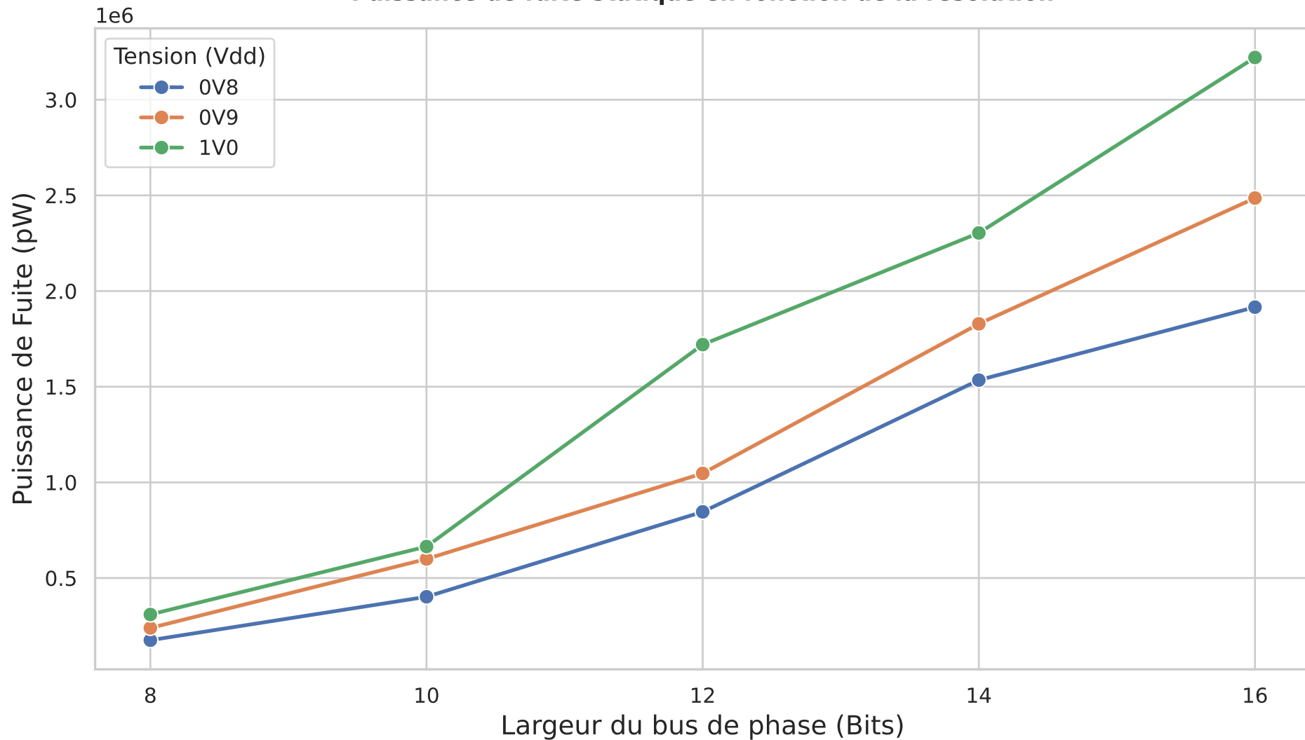
Puissance de fuite statique en fonction de la resolution
