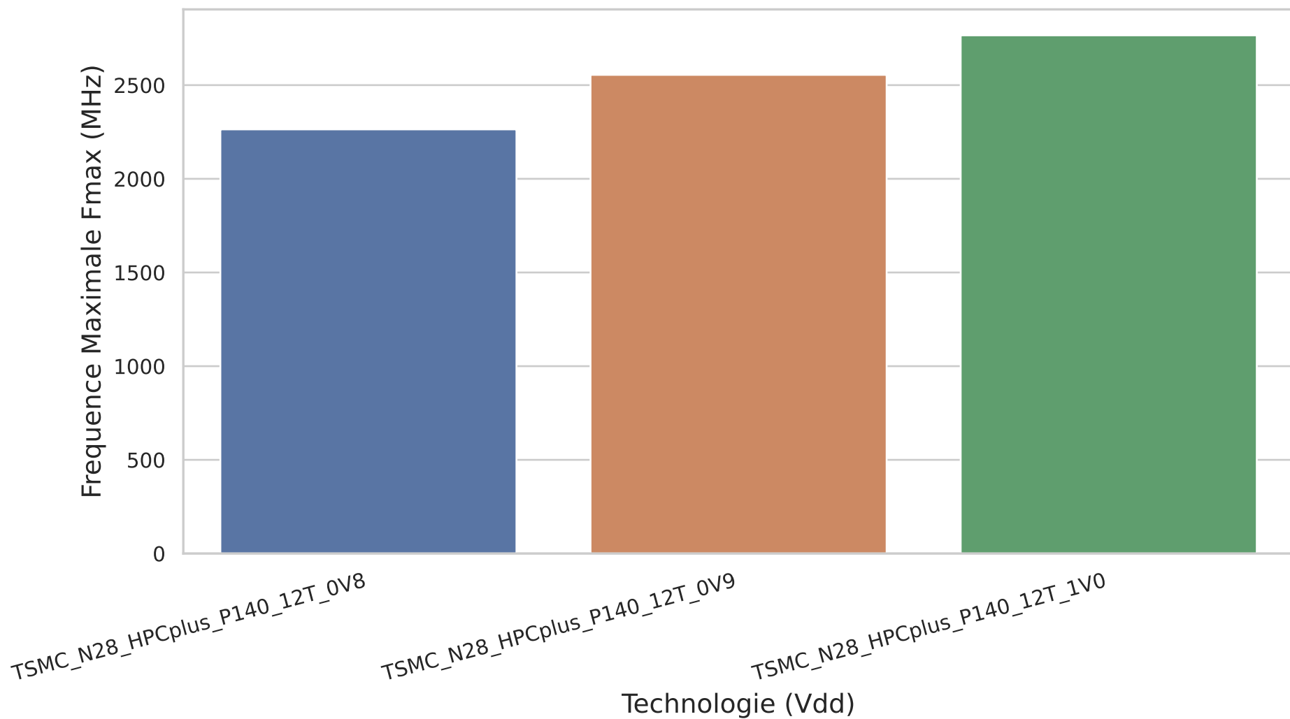
Evolution du Fmax (Bus interne: 22 bits)
