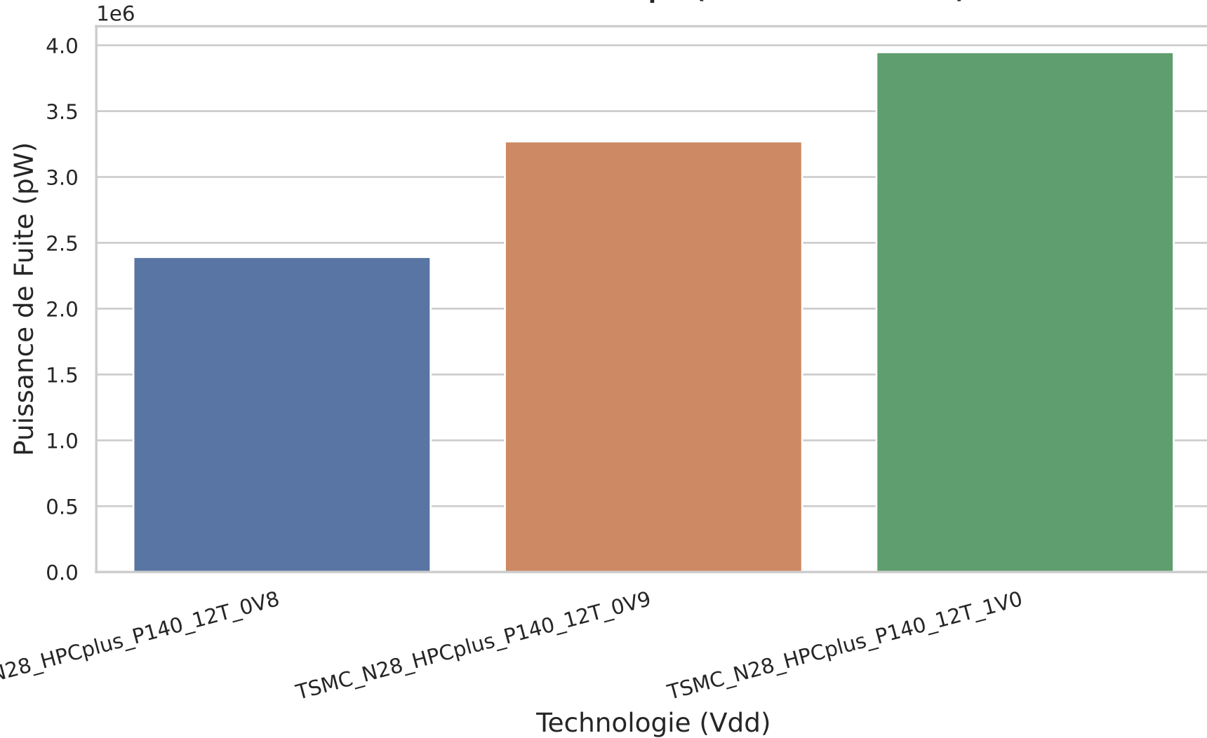
Puissance de fuite statique (Bus interne: 22 bits)
