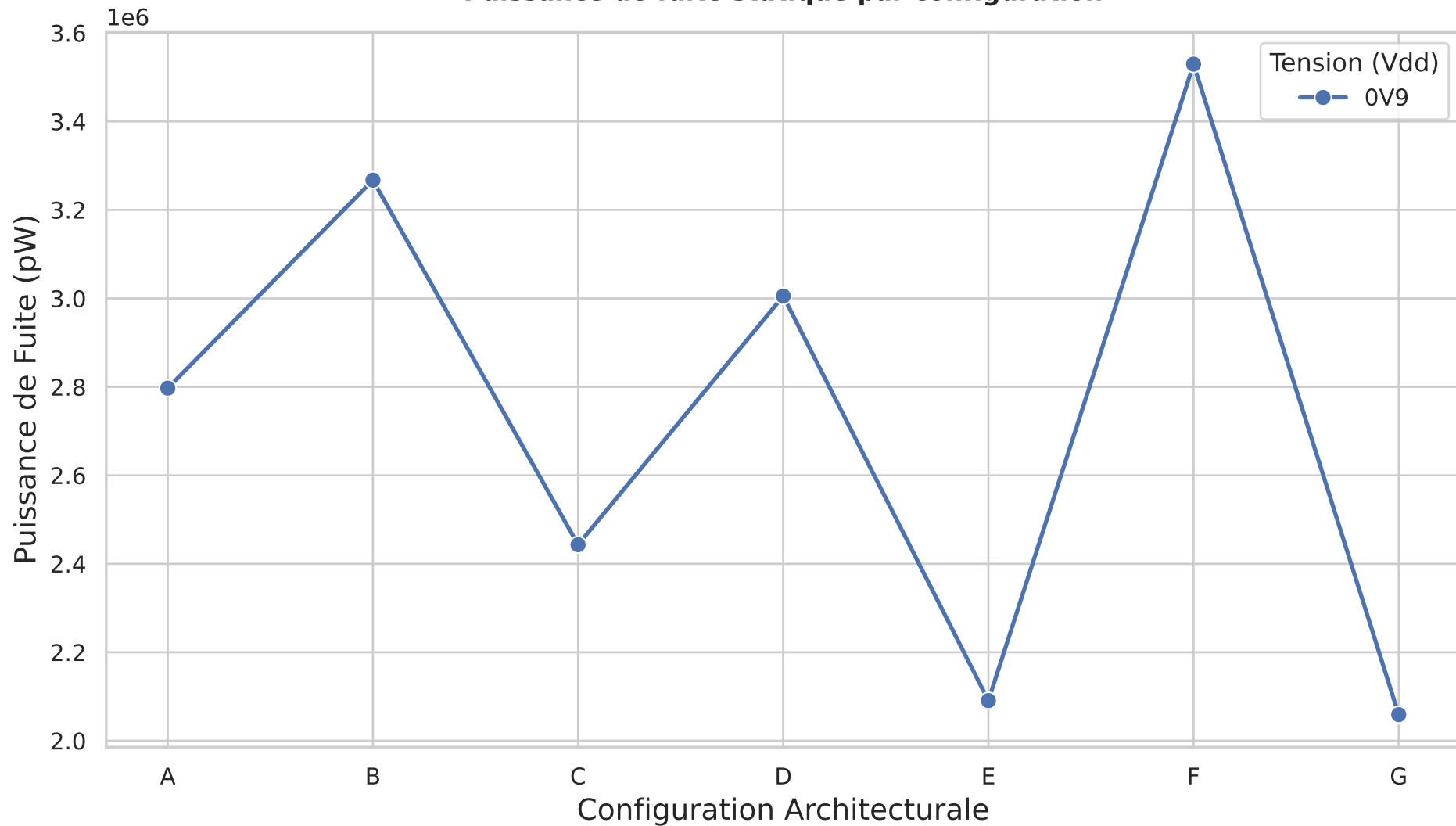
Puissance de fuite statique par configuration
