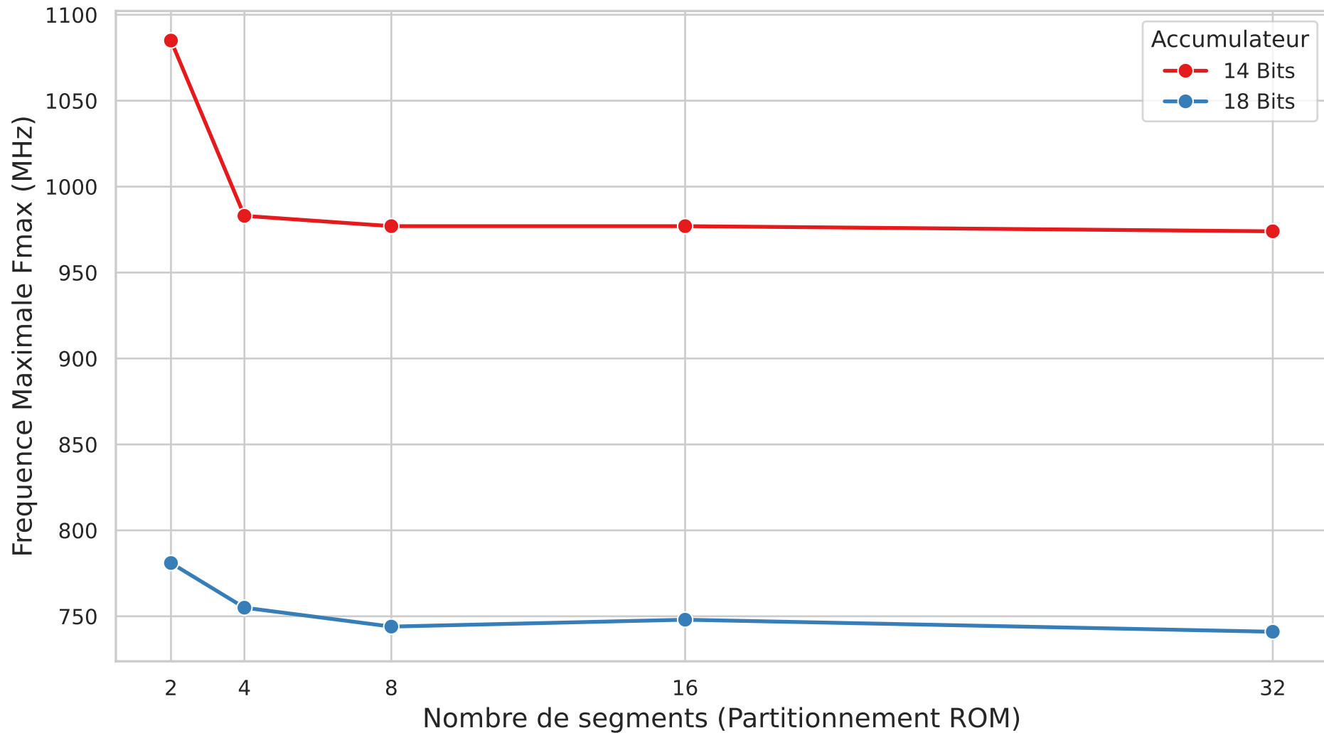
Evolution du Fmax en fonction du nombre de segments
