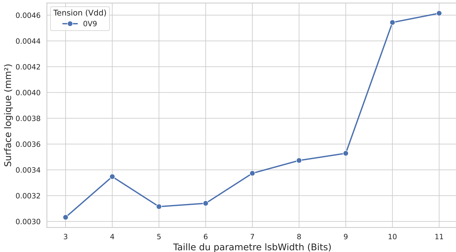
Empreinte silicium en fonction du parametre lsbWidth
